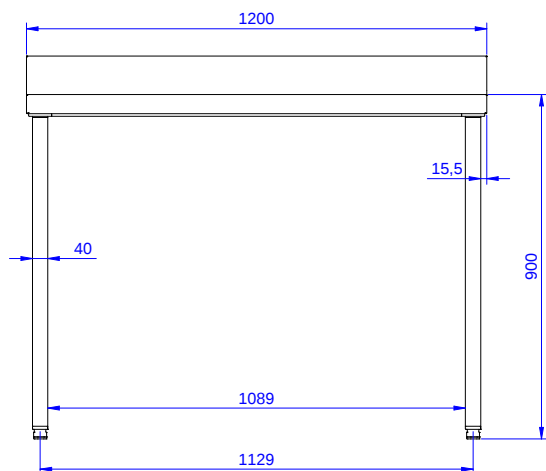
Oldalnézet
